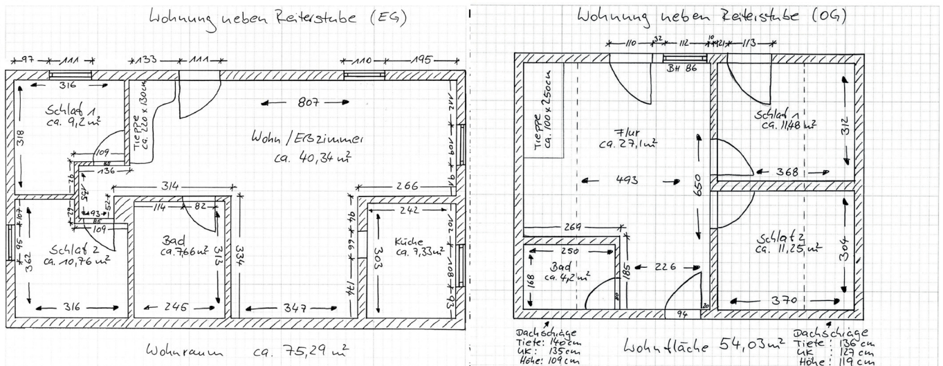
Grundriss Verwalterwohnung ohne Pflegerappartement
